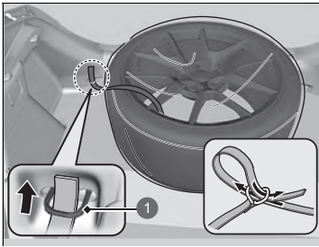
1 Achterste bevestigingspunt
